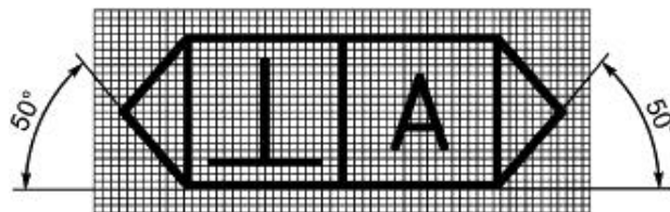
Рисунок С.2 - Знак ориентирующей плоскости
