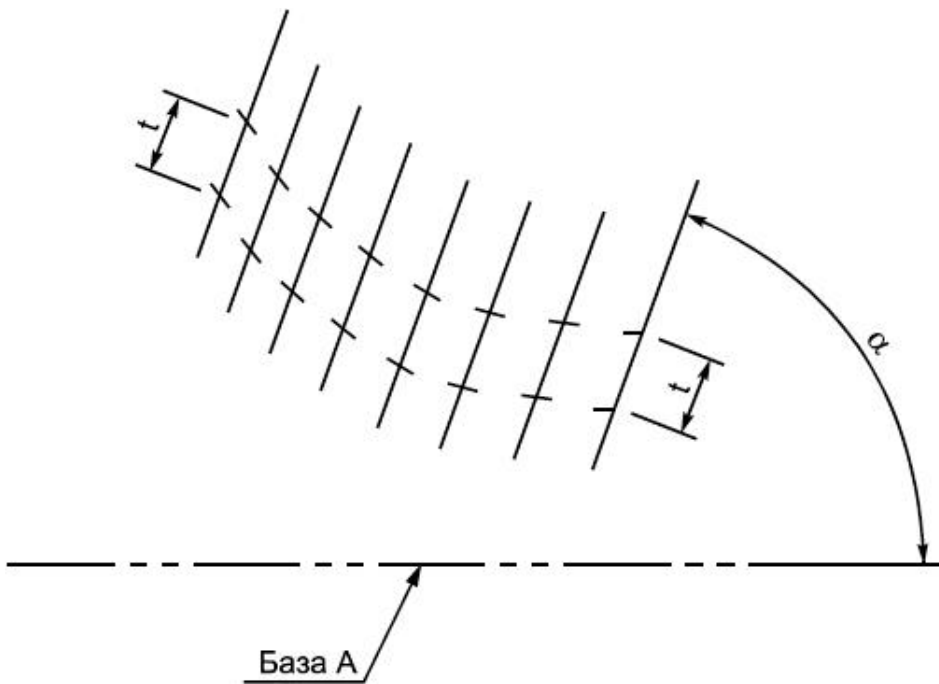
Рисунок 20 - Пояснение к рисунку 19
