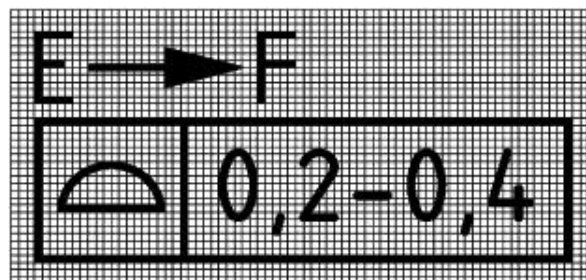
Рисунок С.6 - Знак "от ... до"
