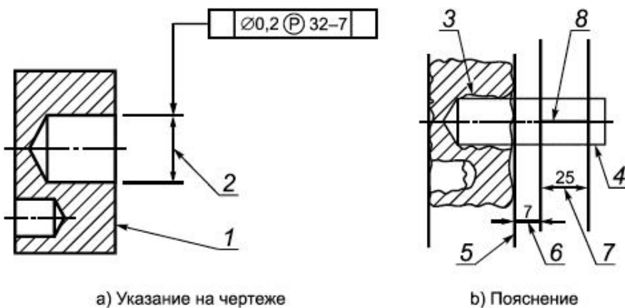
Рисунок 58 - Пример прямого указания смещенного выступающего поля допуска
