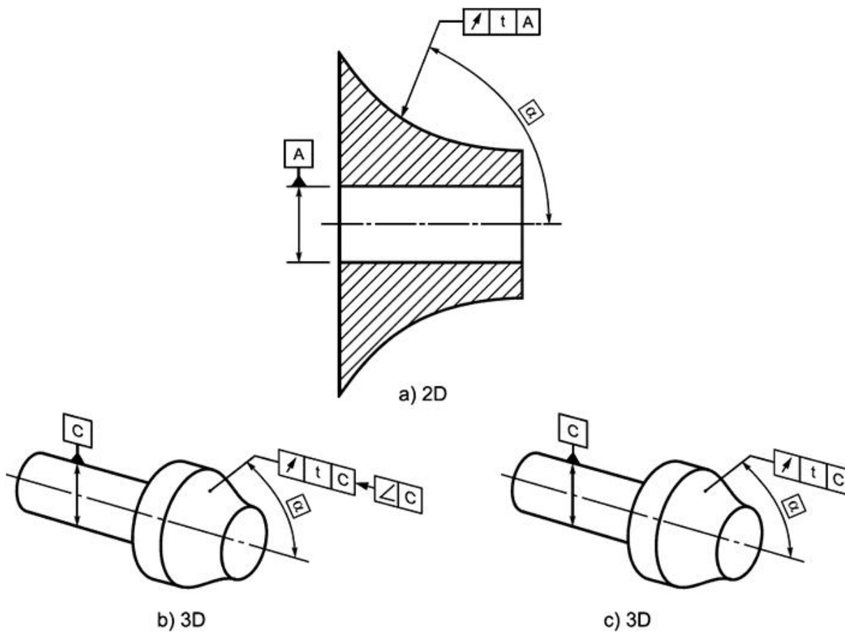
Рисунок 19 - Указание на чертеже
