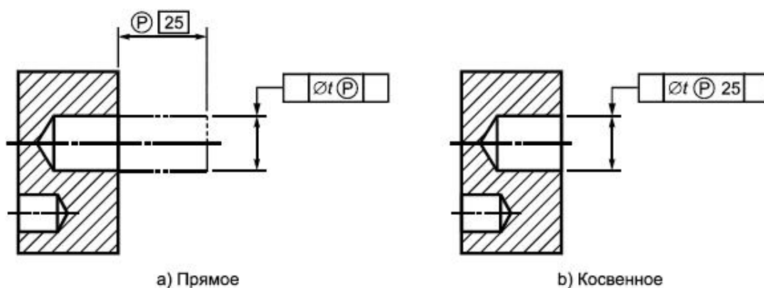
Рисунок 56 - Способы указания выступающего поля допуска
