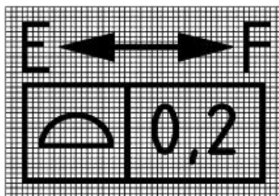
Рисунок С.5 - Знак "между"
