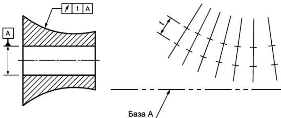
Рисунок 17 - Указание на чертеже Рисунок 18 - Пояснение к рисунку 17
