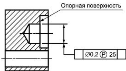
Рисунок 57 - Опорная поверхность выступающего элемента
