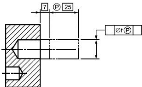
Рисунок 58 - Пример прямого указания смещенного выступающего поля допуска
