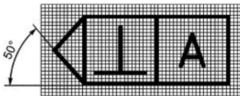
Рисунок С.1 - Знак пересекающей плоскости
