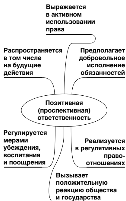
Интеллектуальная карта 14-01
