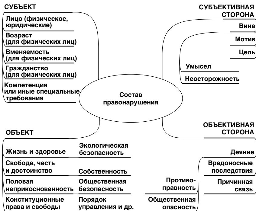
Интеллектуальная карта 13-05
