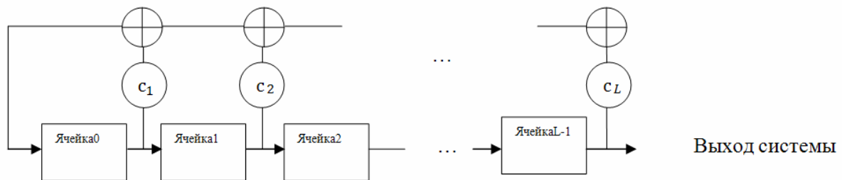
Рисунок 2.2 – Схема операций LFSR.
