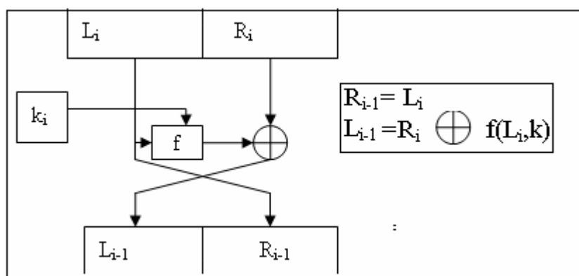
Рисунок 3.7.2 – Обратное преобразование сетью Фейстеля.
